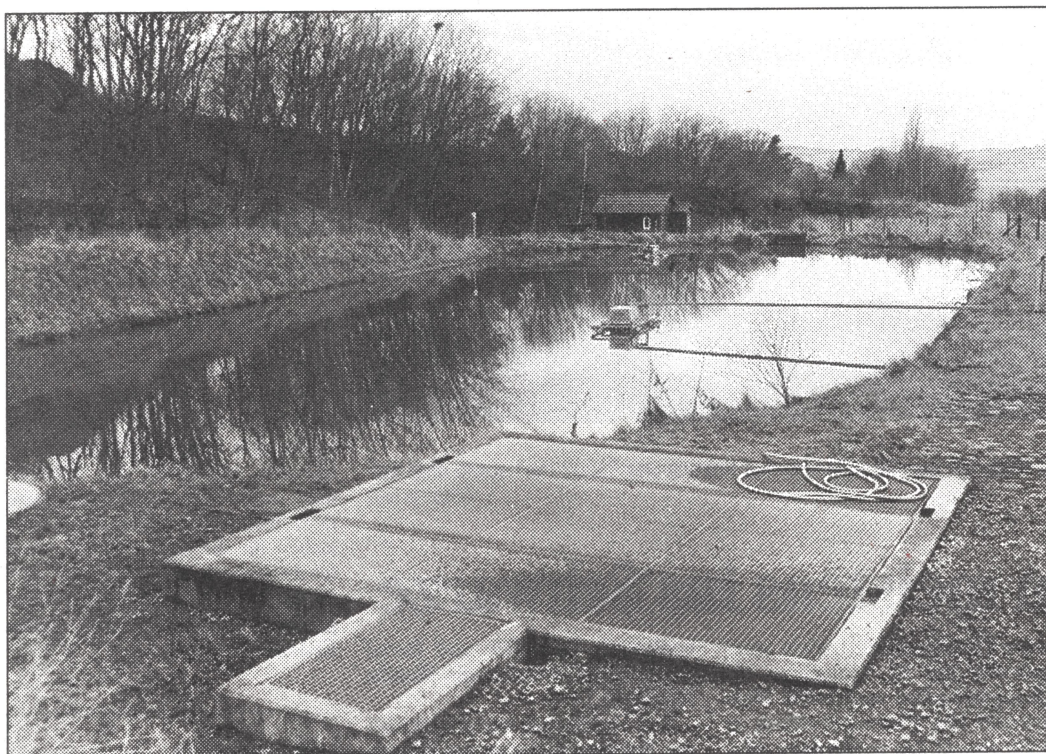
Reileifzen. Brunnenanlage für den Zulauf häuslicher Abwässer. Dahinter der Klärteich.
