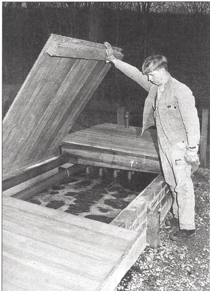
Reileifzen. Der Festbettreaktor in der Teichkläranlage.
